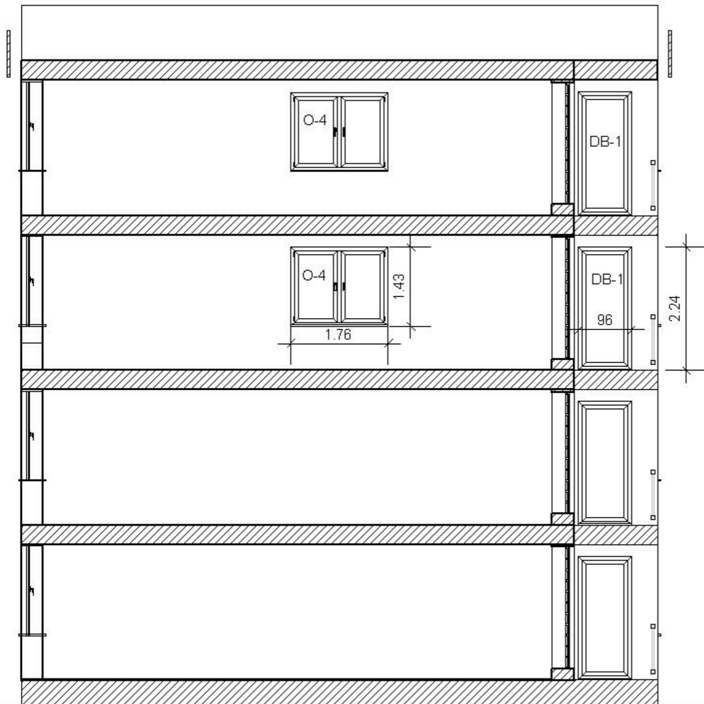
Przekroj przez balkon budynku Internatu 1:100
