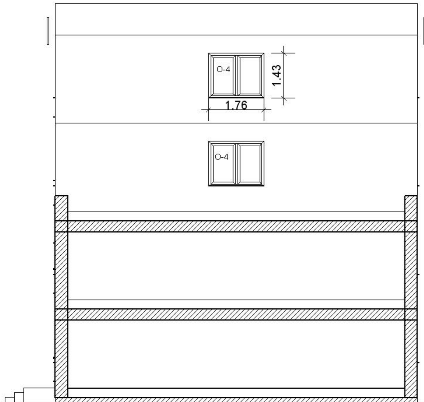
Elewacja boczna budynku Internatu 1:100
