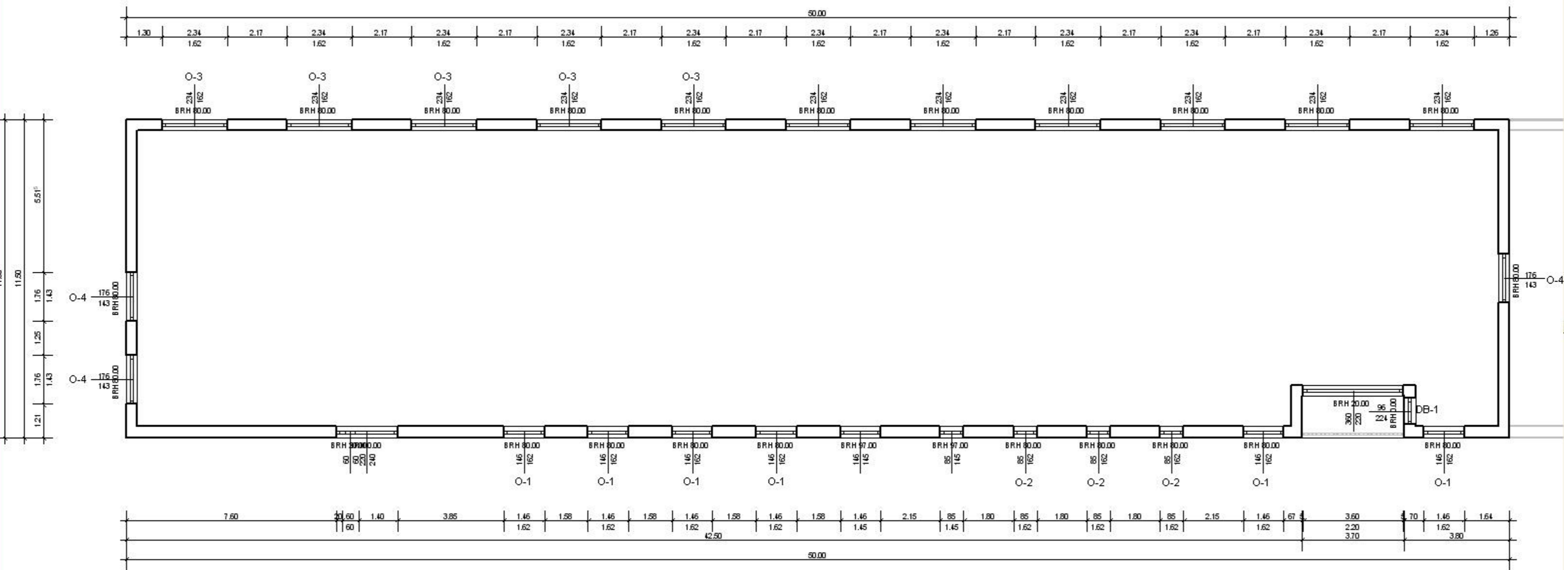
Rzut 2.pietra - budynek Internatu 1:150
